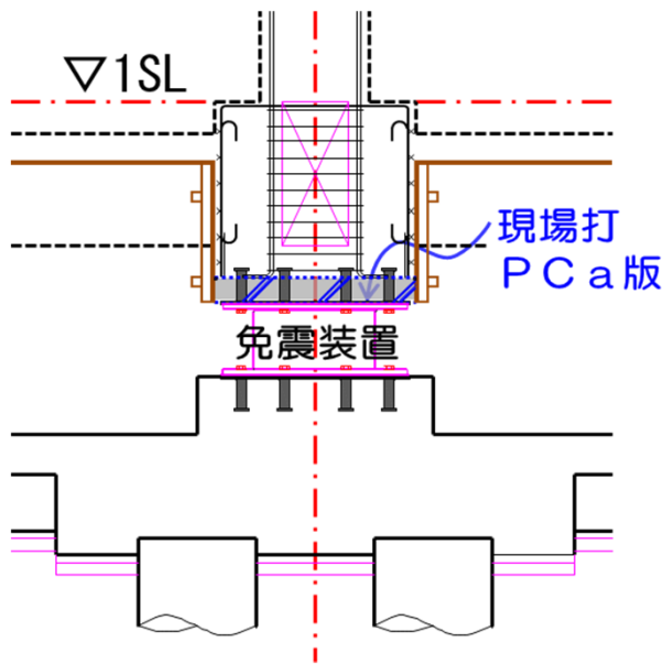
改善案断面図
