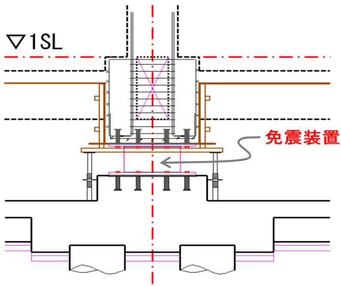
当初計画断面
